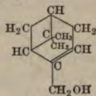
Myrtenol
